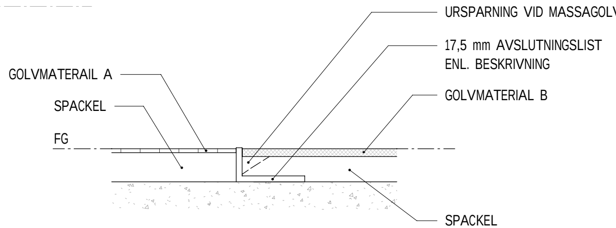
PRINCIPDETALJ MATERIALBYTE GOLV 1 : 2
