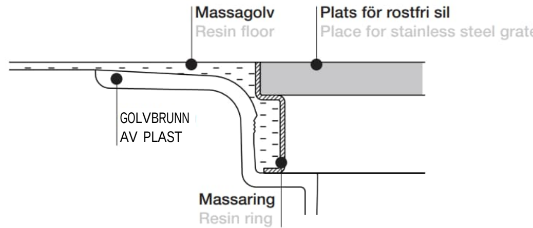
PRINCIPDETALJ GOLVBRUNN AV PLAST I MASSAGOLV ENL. FABRIKANTENS ANVISNING. EJ SKALENLIG
