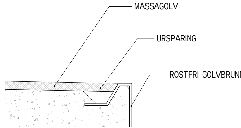
PRINCIPDETALJ RF GOLVBRUNN I MASSAGOLV 1 : 2
